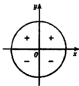
Знаки синуса
