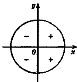
Знаки косинуса
